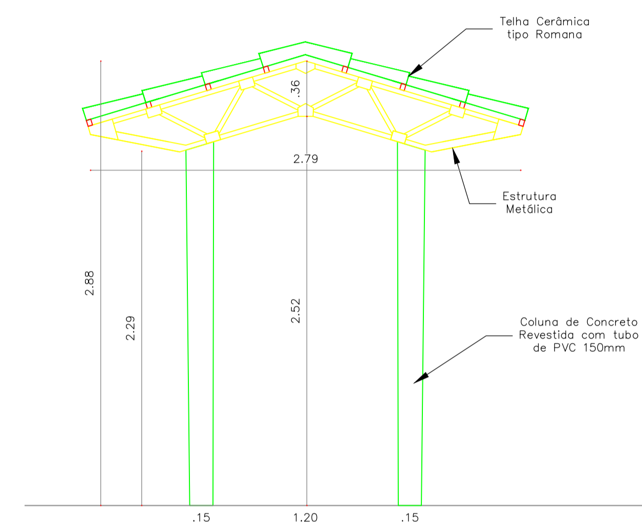
2. DETALHE COBERTA RAMPA Esc.: 1/25
